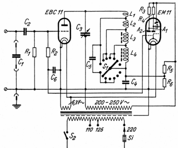
Bild 2. Induskop mit sieben Meßbereichen, mit ungleichgerichtetem Wechselstrom gespeist mit Resonanzanzeige durch eine Abstimmzeigeröhre. C_1 = 400 \text{ pF} ; C_2 = 100 \text{ pF} ; C_3 = 555 \text{ pF} ; C_4 = 50 \text{ nF} ; C_5 = 500 \text{ pF} ; C_6 = 1000 \text{ pF} R_1 = 100 \text{ k}\Omega ; R_2 = 1 \text{ M}\Omega ; R_3 = 1 \text{ M}\Omega ; R_4 = 2 \text{ M}\Omega ; R_5 = 15 \text{ k}\Omega , 2 \text{ W} ; R_6 = 10 \text{ k}\Omega , 2 \text{ W} .
