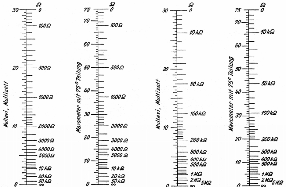
Bild 6. Zahlenleitern zur Umrechnung von Zeigerausschlägen in Ohmwerte. Meßbereich I (Schaltbild 5a).
