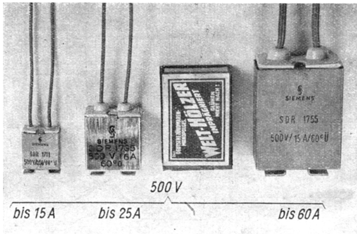
Bild 1. Die neuen Typen der Kleinstdrosselreihe.
