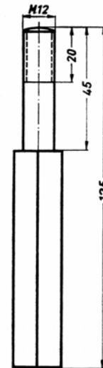
Gewindebolzen
